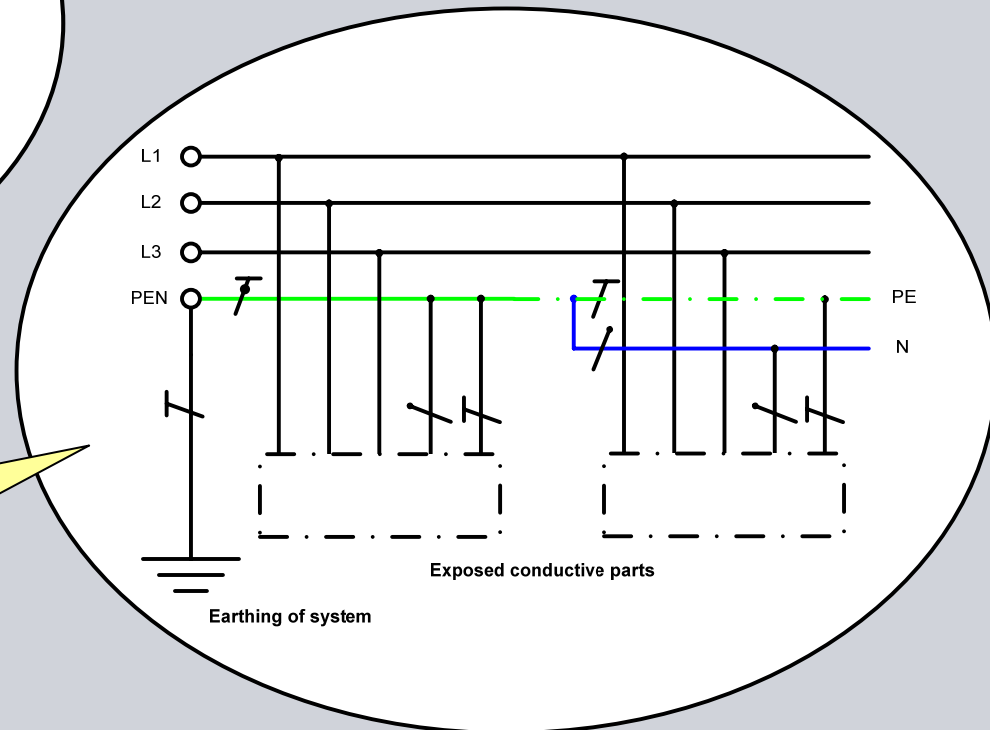
TN-S-System
